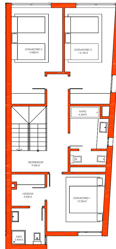
PLANTA PRIMERA 61.00 m2
